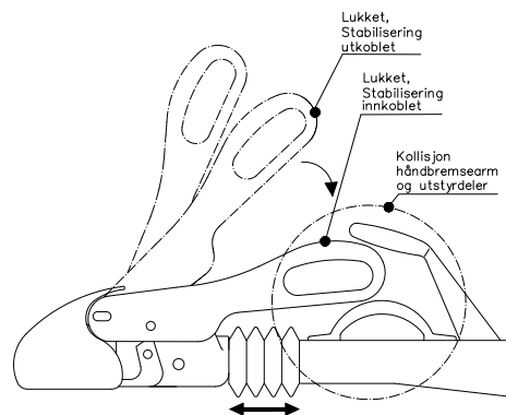
Bilde 5: Slå på stabilisering
