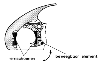
Afbeelding 9: plaatsing van de frictie-elementen
