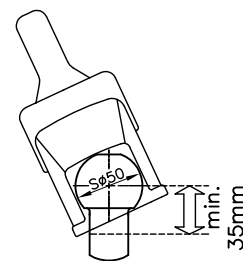
Bilde 1: Kulestang trekkvogn
