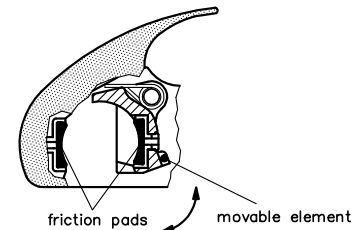
Croquis 9 : Agencement des éléments de friction
