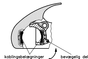
Billede 9: Friktionsbelægningernes anordning
