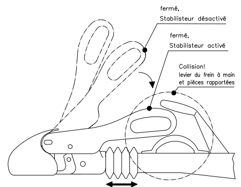
Croquis 5 : Activation de la stabilisation
