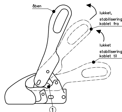
Billede 6: Stabilisering frakobling
