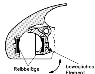
Bild 9: Anordnung der Reibelemente
