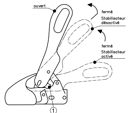
Croquis 6 : Désactivation de la stabilisation Décrochage
