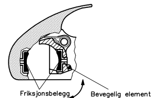
Bilde 9: Anordning for friksjonselementer
