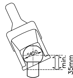
Croquis 1 : Crochet d'attelage véhicule de traction
