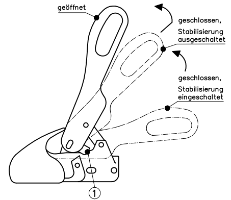
Bild 6: Stabilisierung ausschalten Abkuppeln
