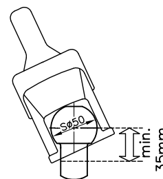
Afbeelding 1: kogelstang trekkend voertuig
