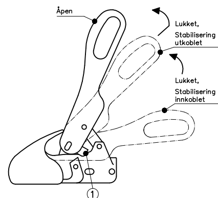
Bilde 6: Slå av stabilisering, frakoble
