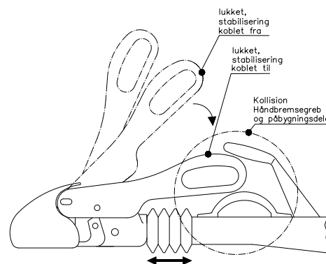
Billede 5: Stabilisering tilkobling
