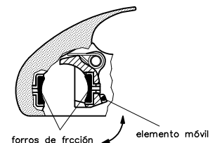
Figura 9: Disposición de los elementos de fricción
