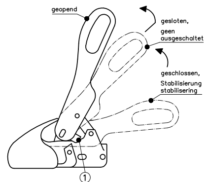
Afbeelding 6: stabilisator uitschakelen loskoppelen
